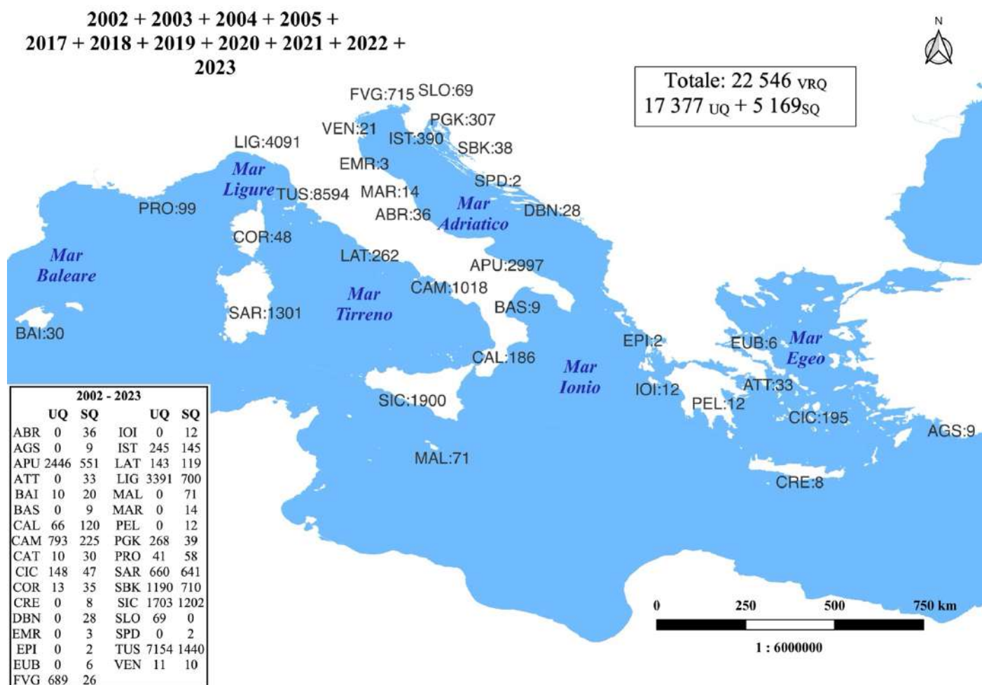
Figura 3. Distribuzione geografica dei questionari appartenenti al fondale roccioso nei due progetti SPA (2002-2005) e DUE (2017- 2023). Il numero totale di schede registrate valide (VQR), mostrato nella mappa per ogni regione, è stato suddiviso in questionari utili (UQ) e questionari scartati (SQ). ABR, Abruzzo; AGS, Agais-Region (Turchia); APU, Puglia; ATT, Attica (Grecia); BAI, Isole Baleari (Spagna); BAS, Basilicata; CAL, Calabria; CAM, Campania; CAT, Catalogna (Spagna); COR, Corsica (Francia); CRE, Creta (Grecia); DBN, Regione raguseo-narentana (Croazia); EMR, EmiliaRomagna; EPI, Epiro (Grecia); EUB, Eubea (Grecia); FVG, Friuli-Venezia Giulia; IOI, Isole Ionie (Grecia); IOC, Santorini (Grecia); IST, Istria (Croazia); LAT, Lazio; LIG, Liguria; MAL, Malta; MAR, Marche; PEL, Peloponneso (Grecia); PGK, Regione litoraneomontana (Croazia); PRO, Provenza (Francia); SAR, Sardegna; SBK, Regione zaratina (Croazia); SIC, Sicilia; SLO, Slovenia; SPD, Regione di Sebenico e Tenin (Croazia); TUS, Toscana; VEN, Veneto.
