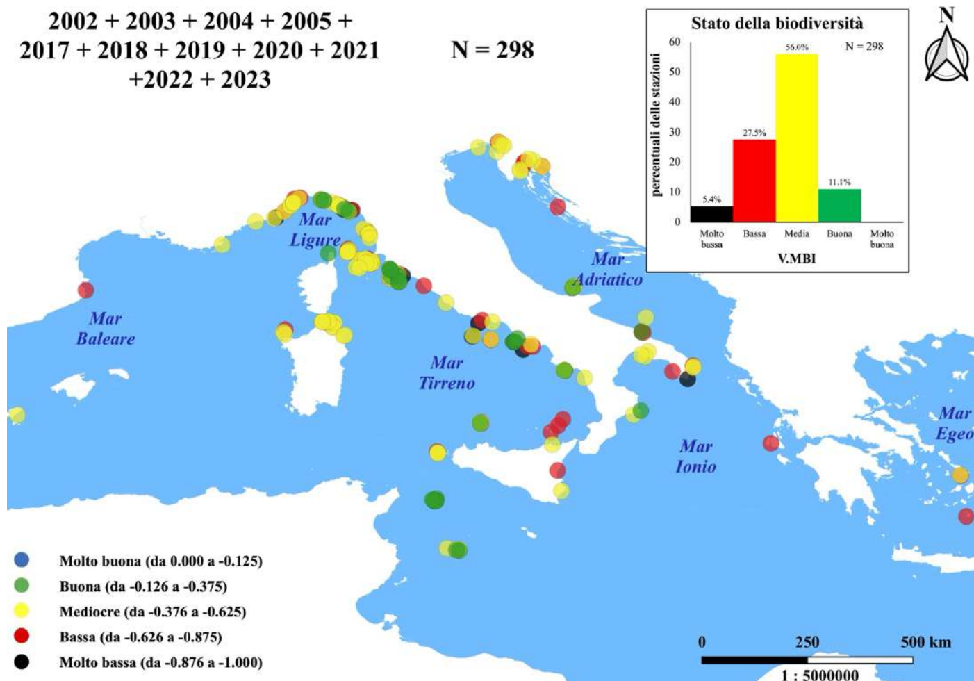
Figura 4. Indice di biodiversità marina (V.MBI) calcolato per le 298 stazioni registrate durante gli 11 anni dei due progetti SPA (2002- 2005) e DUE (2017-2023). Il 56,1% dei siti di immersione ha presentato un punteggio “mediocre”, mentre nessun sito è rientrato nella classe “molto buona”.
