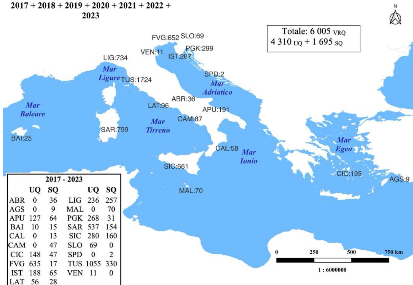
Figura 1. Distribuzione geografica dei questionari appartenenti al fondale roccioso nel progetto di Sentinelle del Mare (2017-2023). Il numero totale di schede registrate valide (VQR), mostrato nella mappa per ogni regione, è stato suddiviso in questionari utili (UQ) e questionari scartati (SQ). ABR: Abruzzo; AGS: Agais-Region (Turchia); APU: Puglia; BAI: Isole Baleari (Spagna); CAL: Calabria; CAM: Campania; EMR: Emilia-Romagna; FVG: Friuli-Venezia Giulia; GRE: Grecia; IST: Istria (Croazia); LAT: Lazio; LIG: Liguria; MAL: Malta; PGK: Regione litoraneomontana (Croazia); SAR: Sardegna; SIC: Sicilia; SLO: Slovenia; SPD: Regione di Sebenico e Tenin (Croazia); TUS: Toscana; VEN: Veneto.
